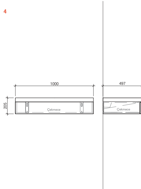
Çekmeceli Bench 100 cm Ön ve Yan Görünüş
