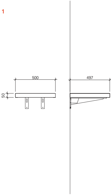
Bench 50 cm Ön ve Yan Görünüş
