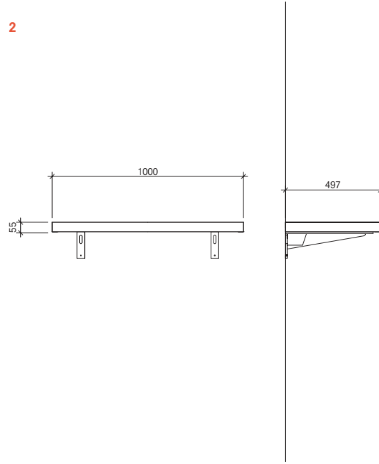
Bench 100 cm Ön ve Yan Görünüş
