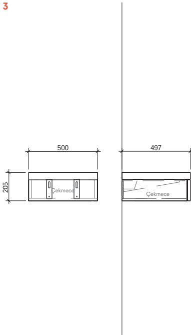
Çekmeceli Bench 50 cm Ön ve Yan Görünüş
